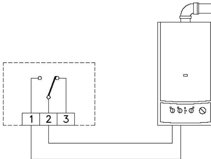
Рис. 4 Схема соединения
